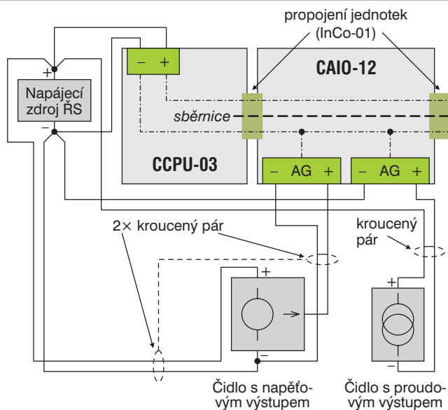
Napájení aktivních čidel ze společného zdroje
