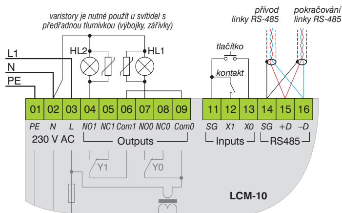
Obr. 4: Příklad svorkového připojení modulu LCM-10
