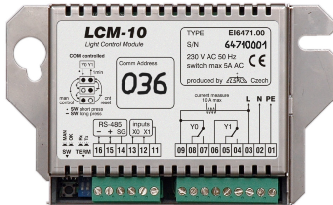
Obr. 1: Pohled na modul LCM-10
