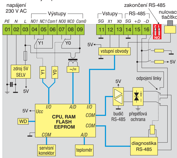
Obr. 2: Vnitřní blokové schéma LCM-10
