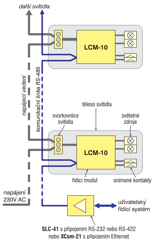
Obr. 3: Příklad zapojení modulů LCM-10 pro řízení řady svítidel
