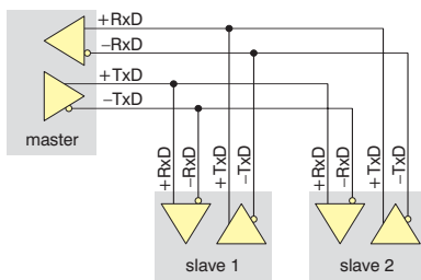
Obr. 13. Vícebodová síť RS-422
