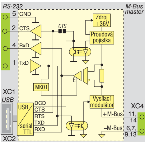
Obr. 28: Převodník s modulem PMBUS/M (EI6011/6012.80) s automat. řízením přijímače
