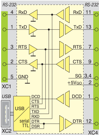
Obr. 6. Převodník s modulem P232GPE (EI6011/6012.50)
