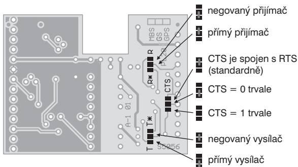
Obr. 23. Propojky na modulu PL20GPS
