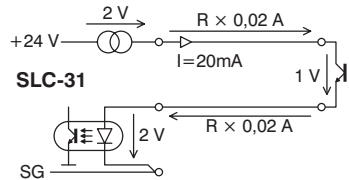
Obr. 27: Rozložení úbytků napětí na vedení
