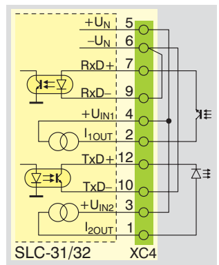
Obr. 26. Různá zapojení aktivního vysíláče a přijímače
