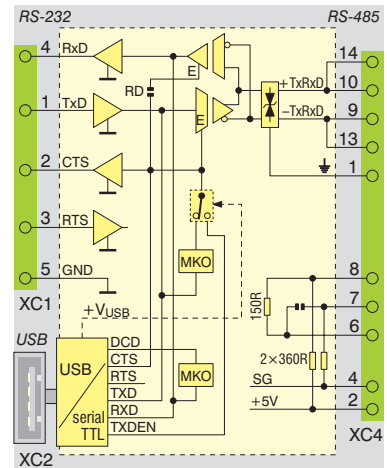
Obr. 18. Převodník s modulem P485GPE, automatické řízení vysíláče od signálu Tx/D
