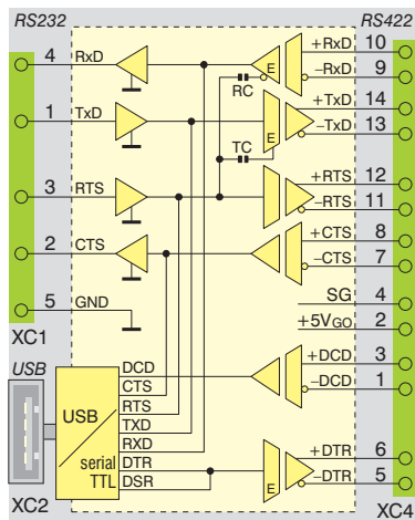
Obr. 11. Převodník s modulem P422GPE pro duplexní provoz (EI6011/6012.20)
