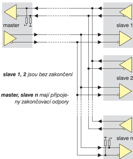
Obr. 14: Zakončení vícebodové sítě RS-422
