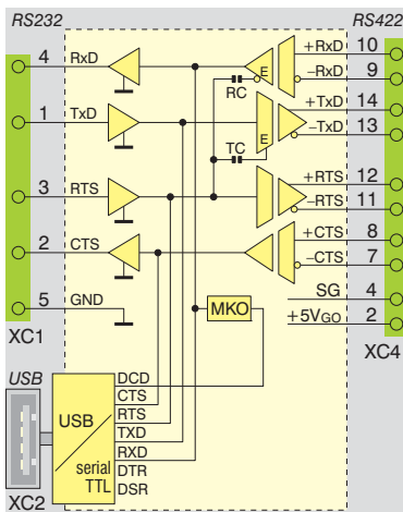
Obr. 10. Převodník s modulem P422GPS pro duplexní provoz (EI6011/6012.30)
