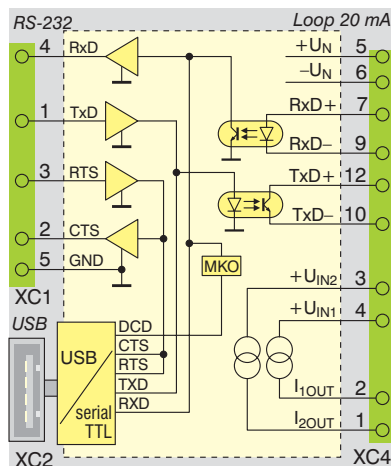
Obr. 22. Převodník s modulem PL20GPS (EI6011/6012.70)
