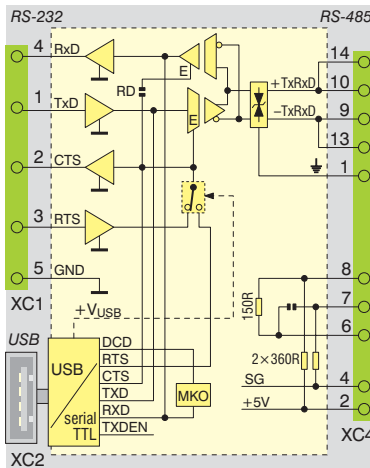
Obr. 17. Převodník s modulem P485GPE, řízení vysíláče RTS (EI6011/6012.40)
