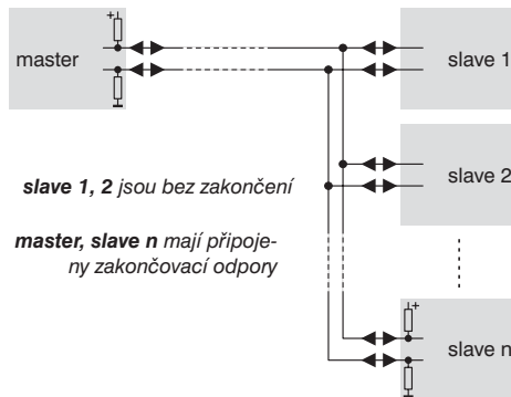
Obr. 21: Zakončení sítě RS-485
