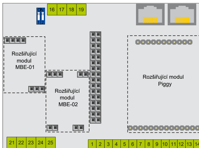
Rozložení rozšiřujících modulů na spodní desce XCOM-33
