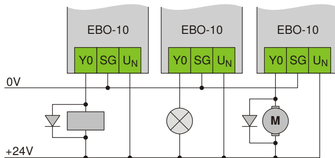
Obr. 10: Způsob připojení zátěže k EBO-10
