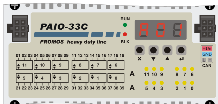
Obr. 13: Přední panel PAIO-33C
