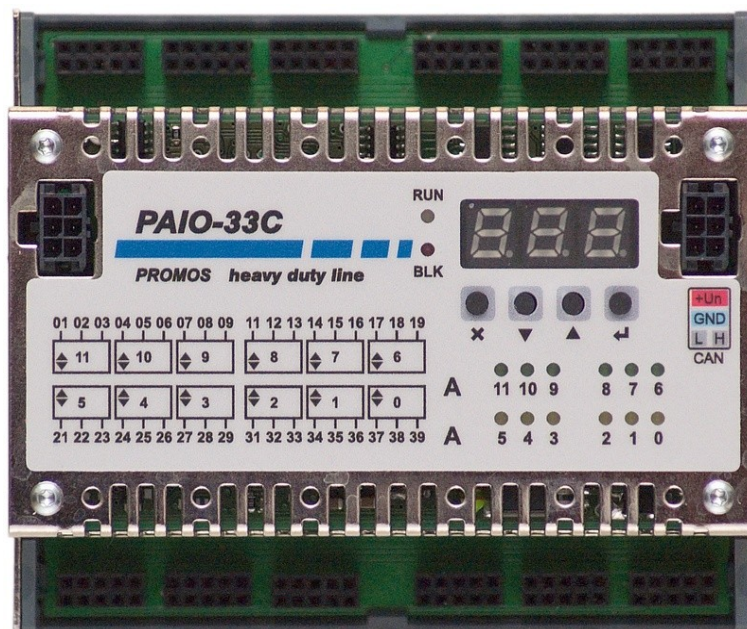
Obr. 1: Jednotka PAIO-33C
