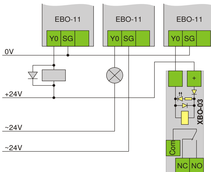
Obr. 12: Způsob připojení DC zátěže k EBO-11
