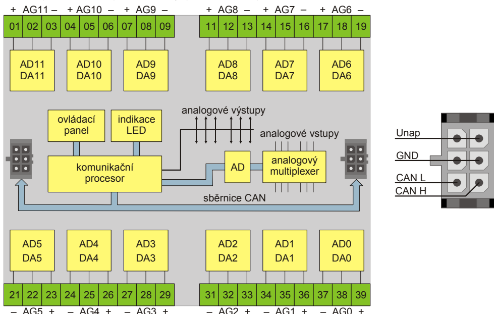
Obr. 2: Blokové schéma jednotky PAIO-33C
