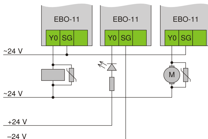
Obr. 11: Způsob připojení AC zátěže k EBO-11
