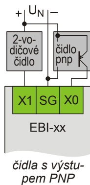
Obr. 9: Připojení binárních vstupů
