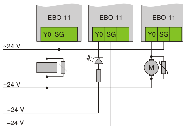
Obr. 11: Způsob připojení AC zátěže k EBO-11
