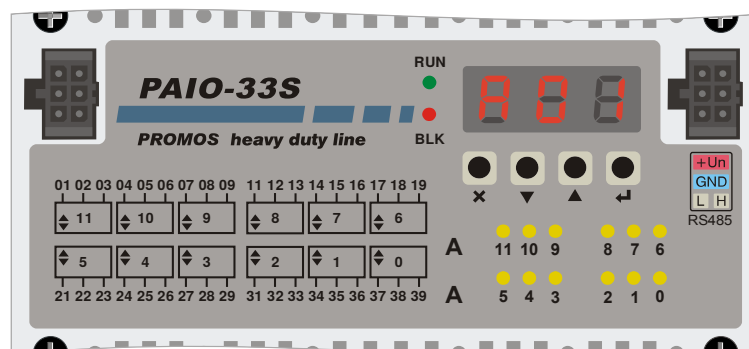
Obr. 13: Přední panel PAIO-33S
