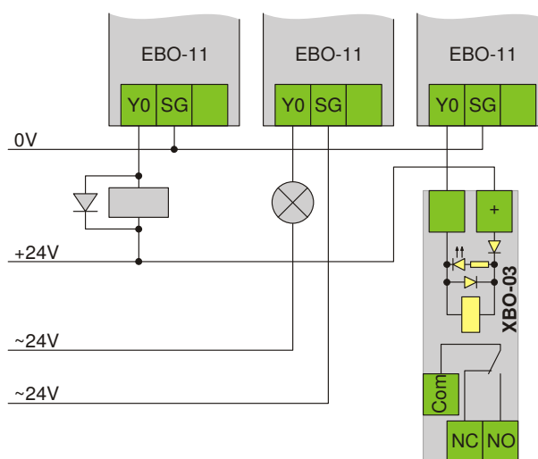
Obr. 12: Způsob připojení DC zátěže k EBO-11
