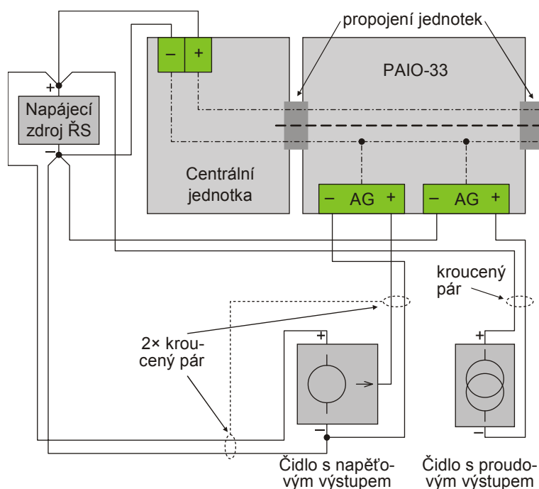
Obr. 5: Čidla napájená ze zdroje řídicího systému
