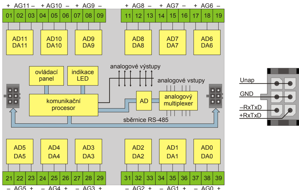
Obr. 2: Blokové schéma jednotky PAIO-33S
