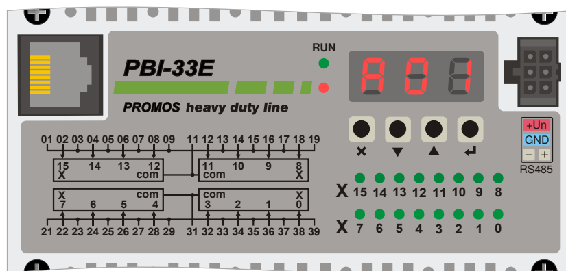
Obr. 8: Přední panel PBI-33E
