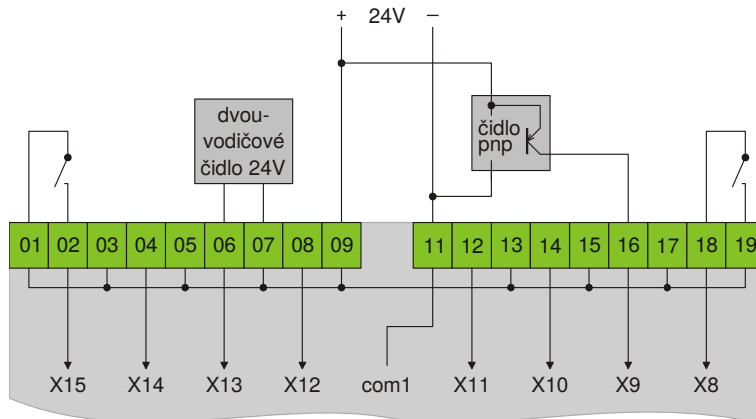
Obr. 4: Připojení čidel pnp ke vstupům PBI-33E
