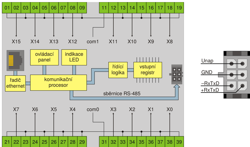
Obr. 2: Blokové schéma jednotky PBI-33E
