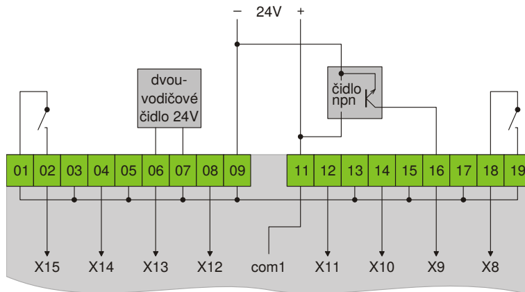
Obr. 3: Připojení čidel npn ke vstupům PBI-33E
