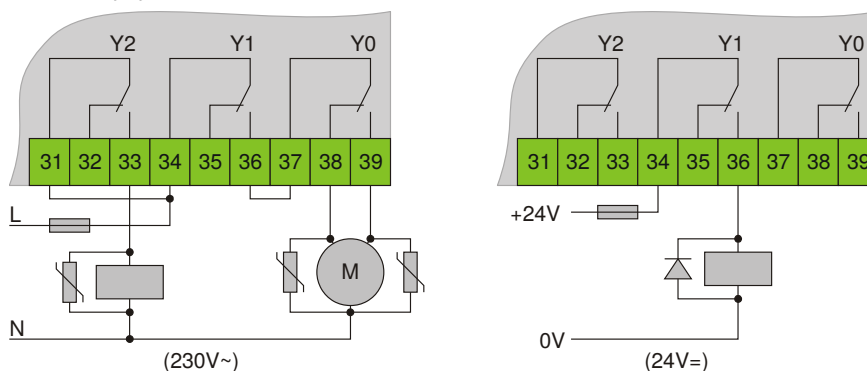
Obr. 3: Ošetření připojení indukční zátěže k PBO-33E
