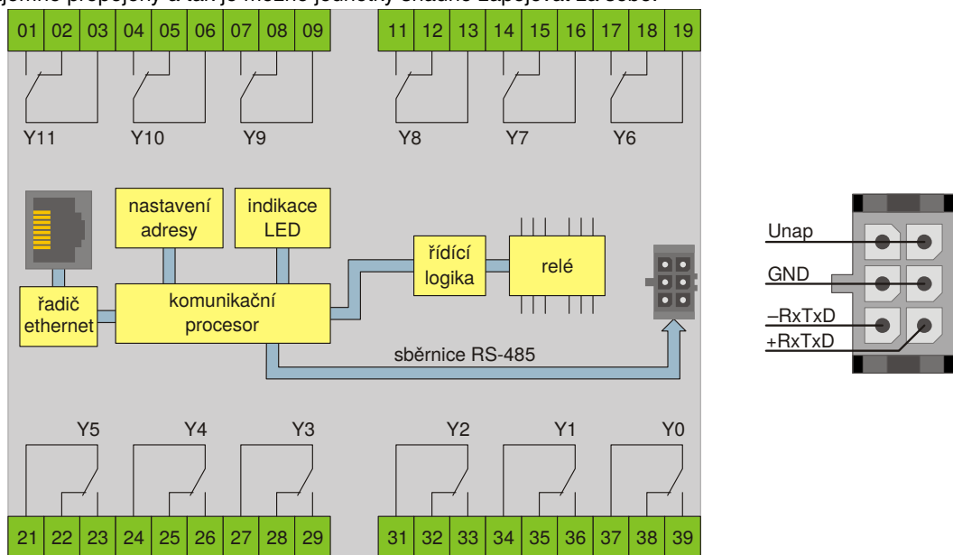
Obr. 2: Blokové schéma jednotky PBO-33E
