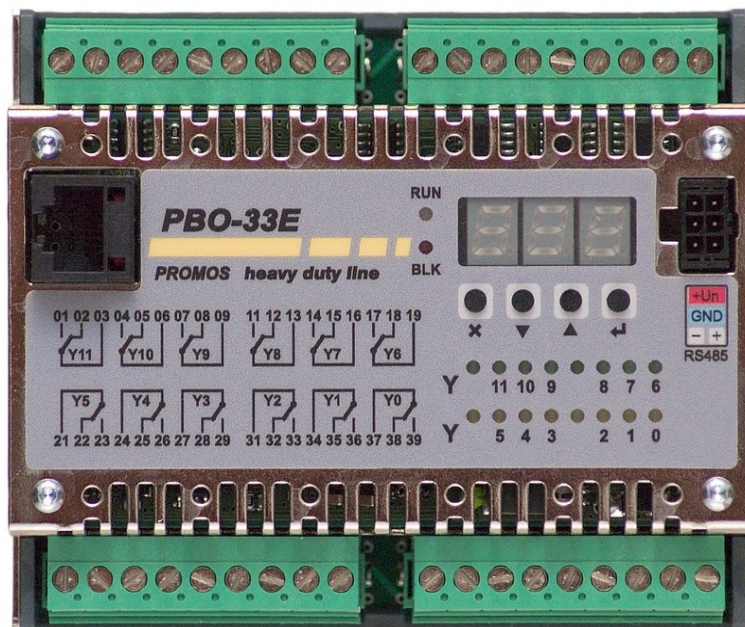
Obr. 1: Jednotka PBO-33E
