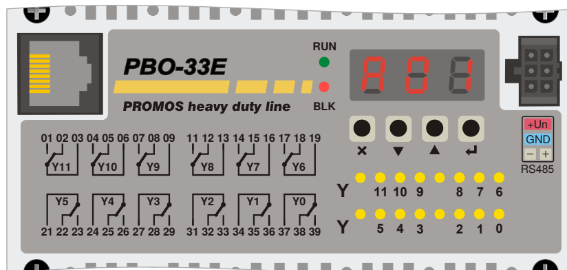
Obr. 4: Přední panel PBO-33E
